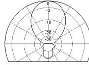
[水平偏波・水平面]
