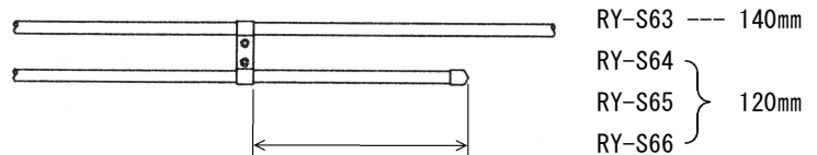
[図 4] ショートバーの位置 (出荷時組付済)
